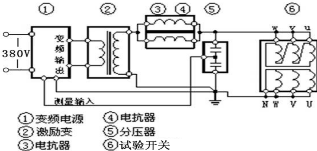
开关试验接线图
