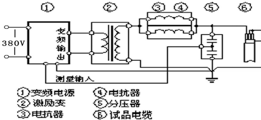
电缆耐压试验接线图
